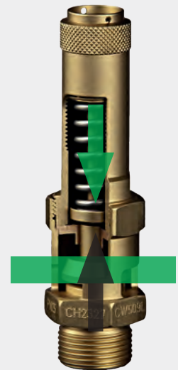
Ventil ist geöffnet F_s < F_p
