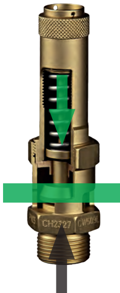
Ventil ist geschlossen F_s > F_p
